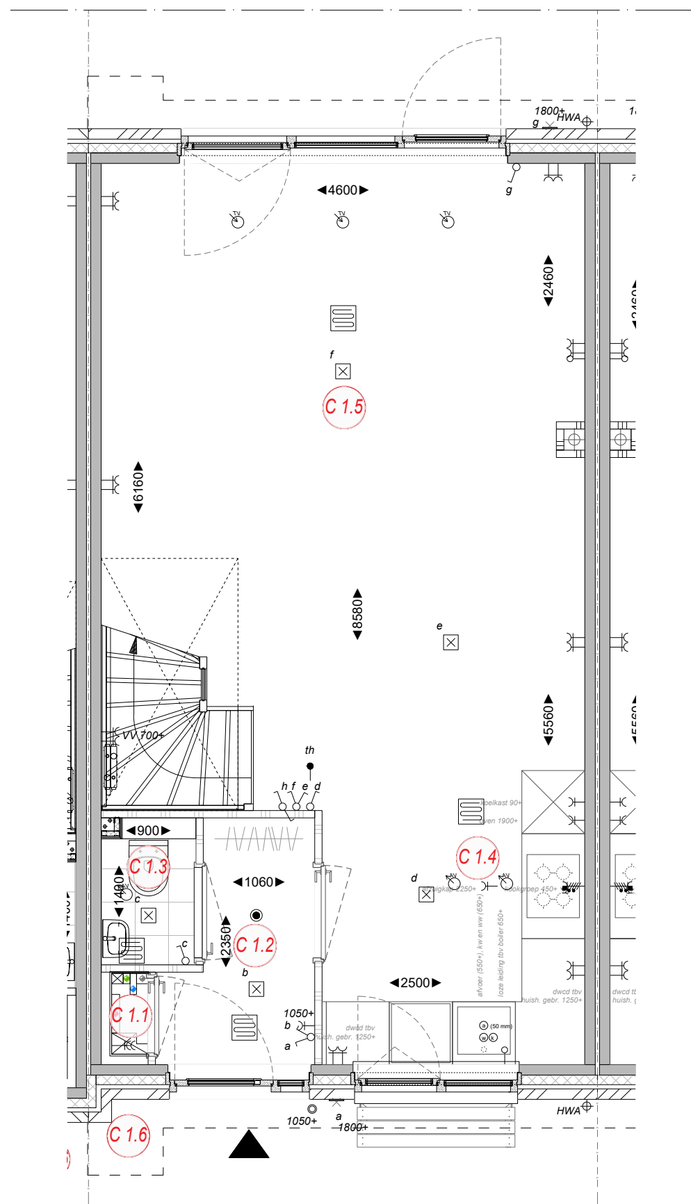
Begane grond
