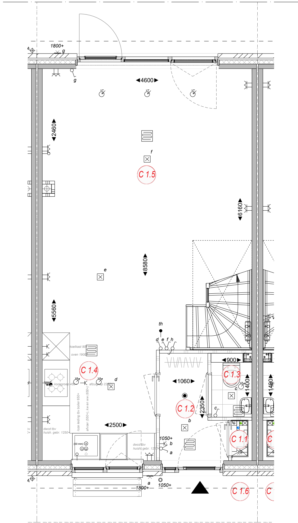
Begane grond
