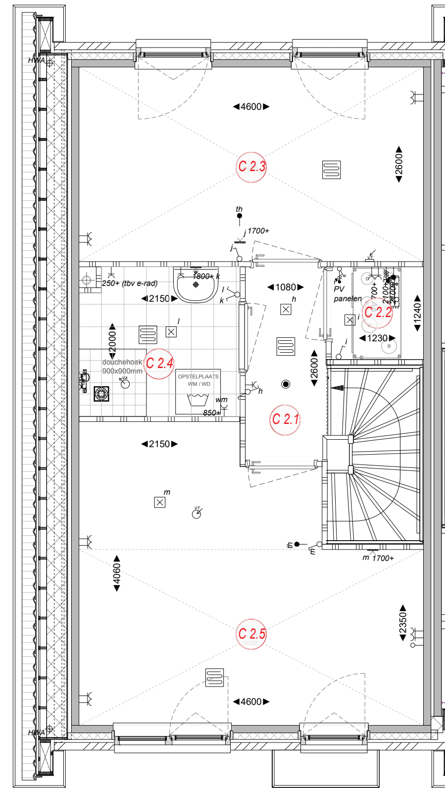
Eerste verdieping
