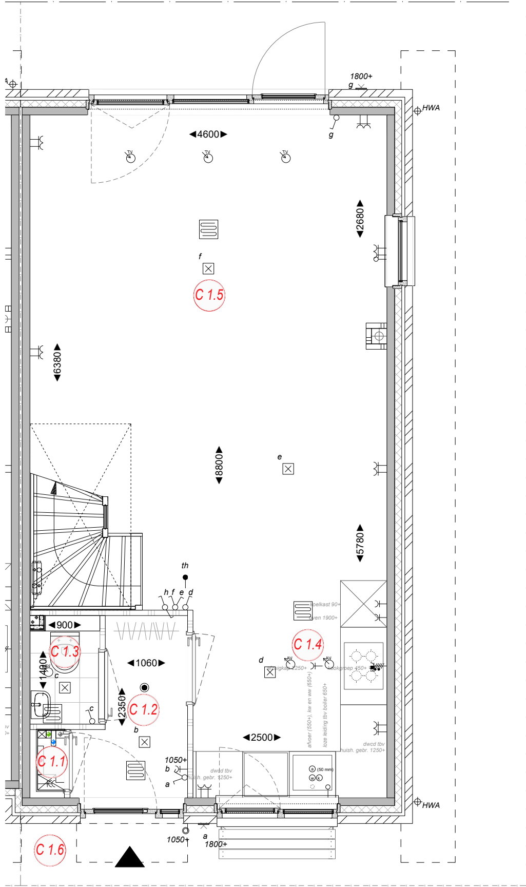
Begane grond
