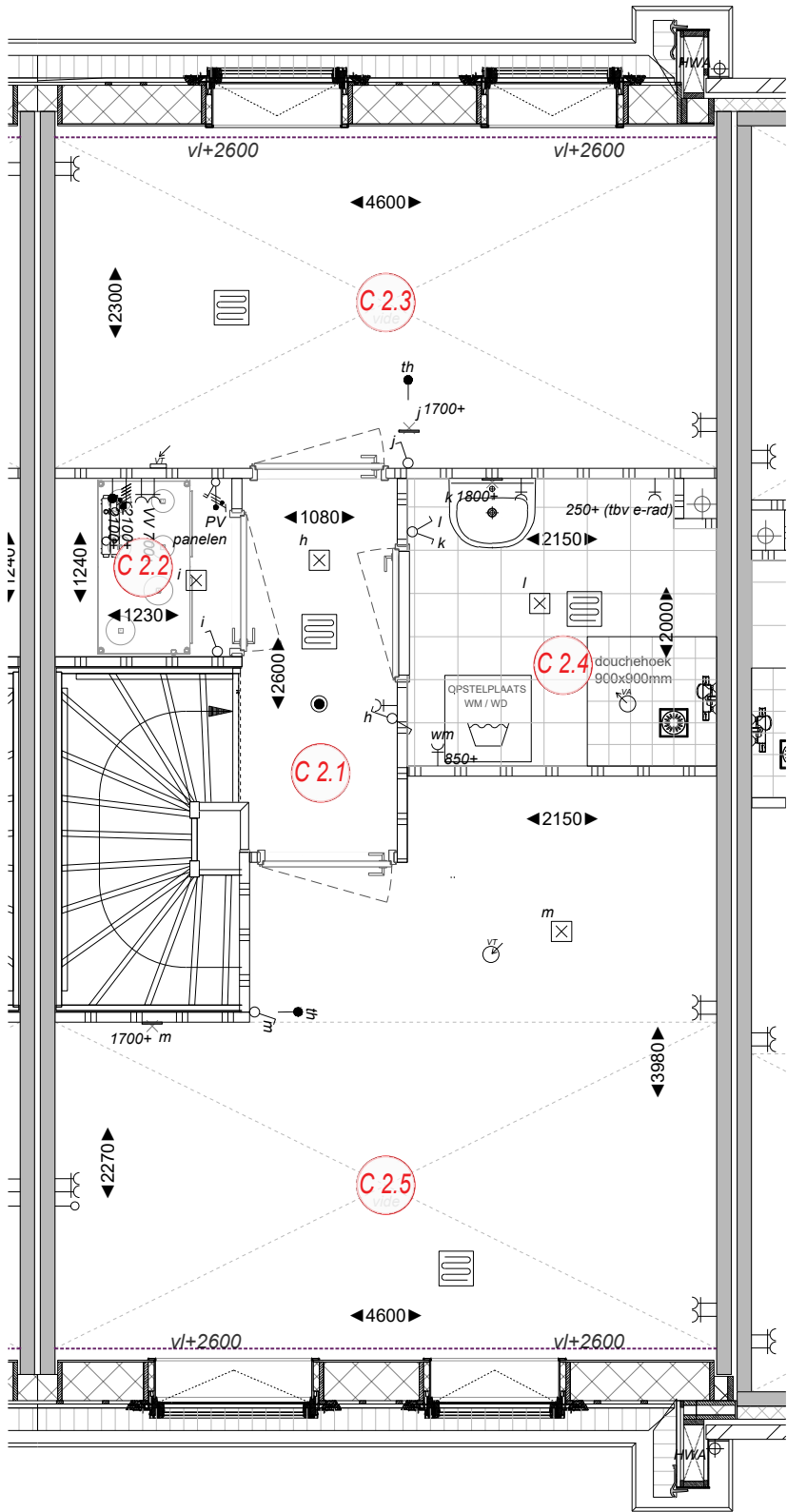
Eerste verdieping
