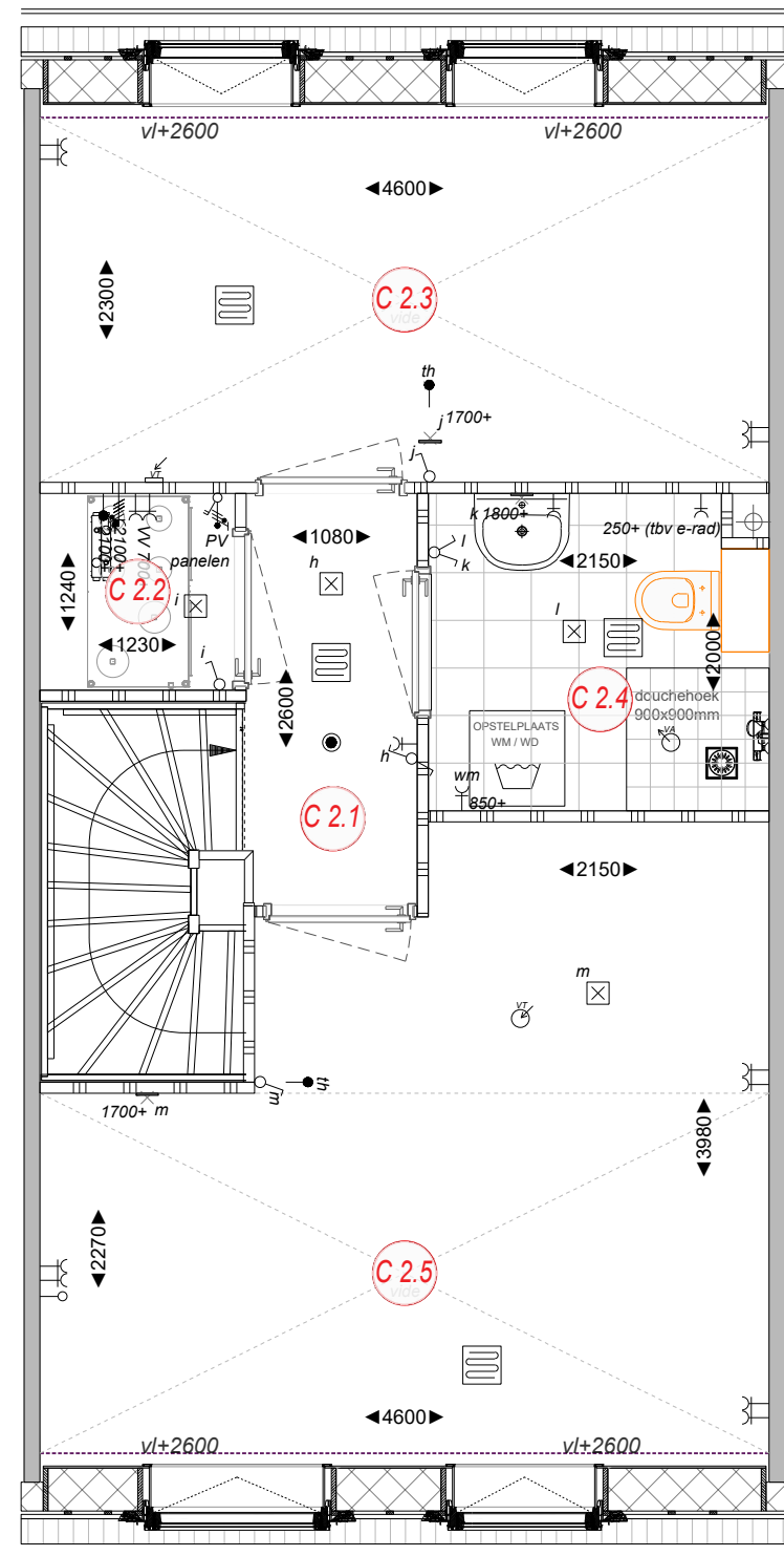
Tussenwoning
