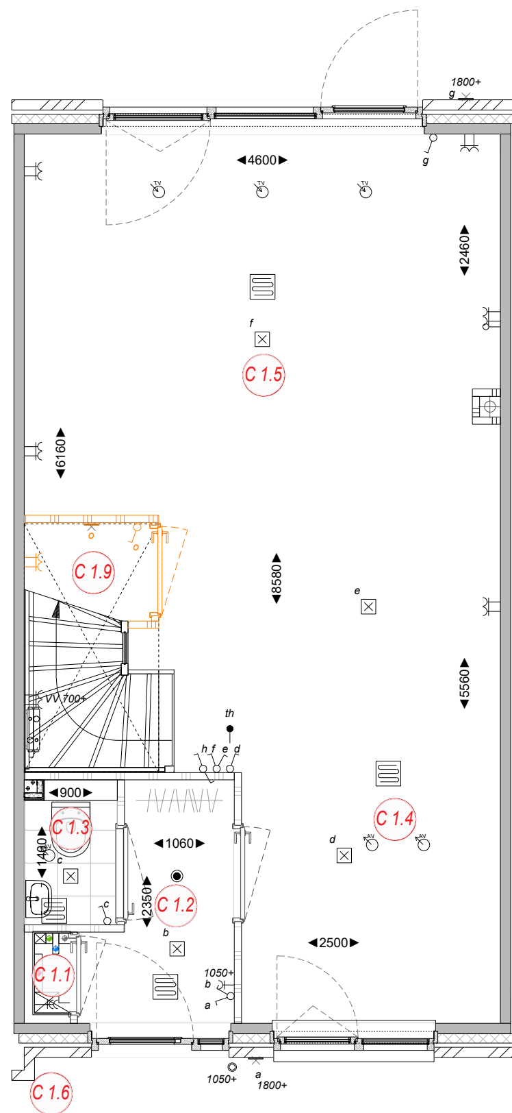
Tussenwoning
