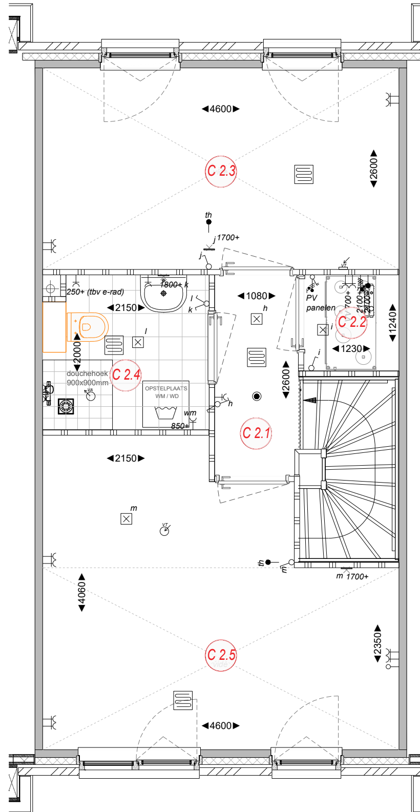
Kopwoning
