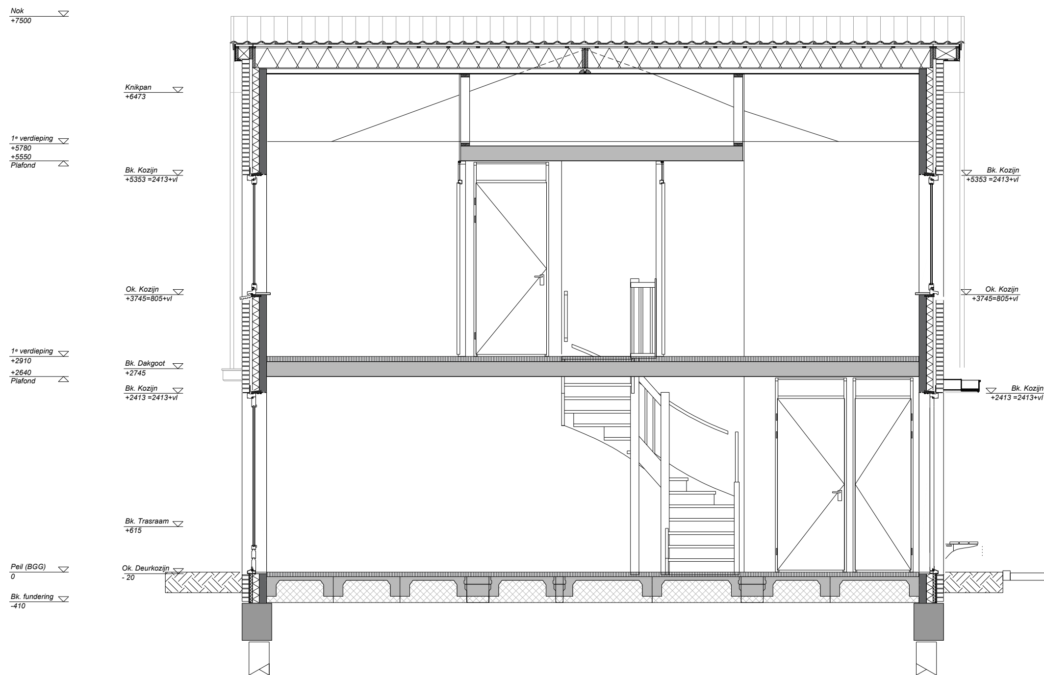
Doorsnede kopwoningen
