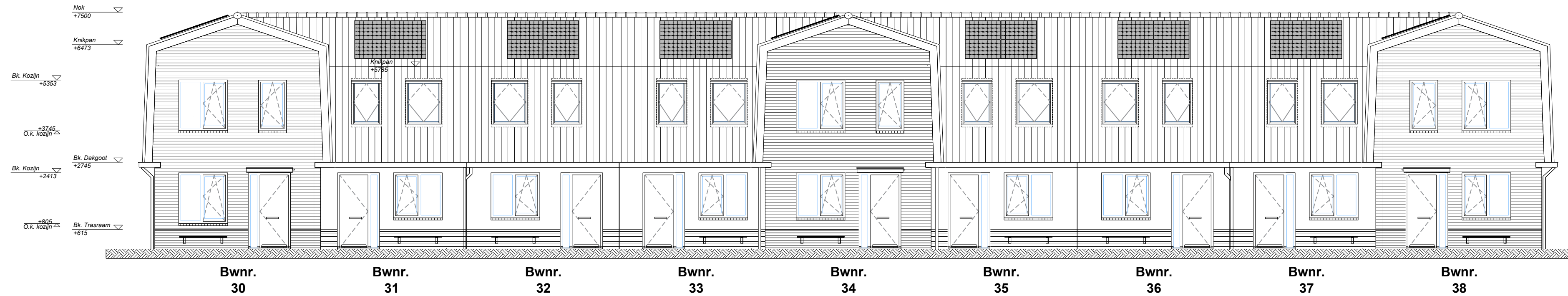
Voorgevel
