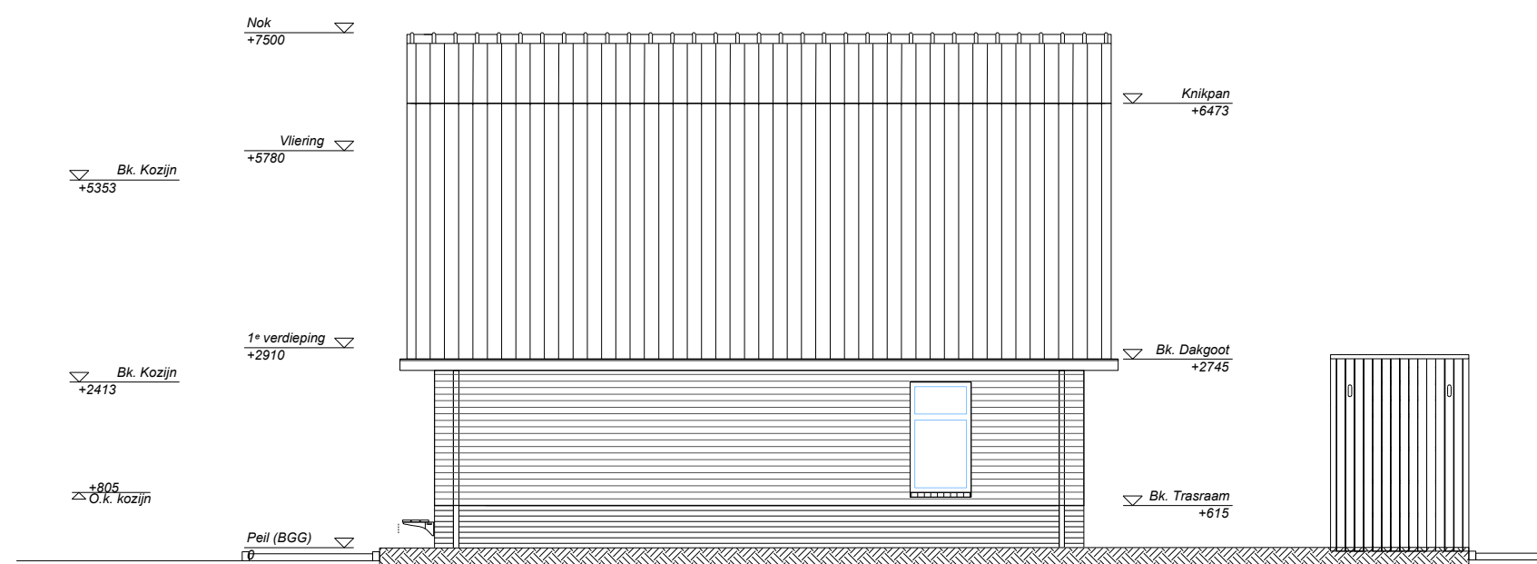
Zijgevel
