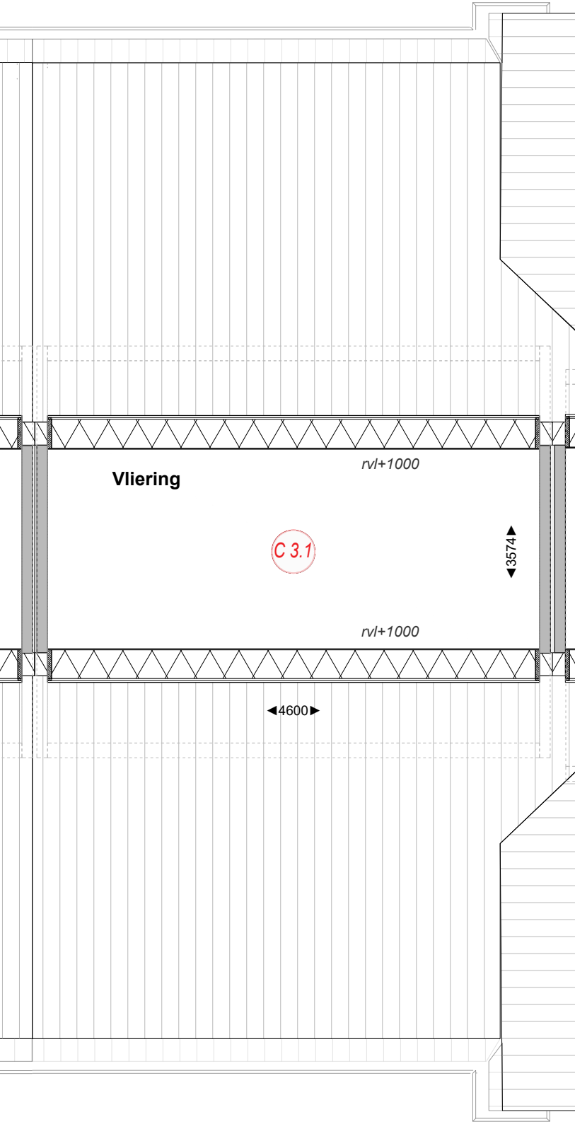
Vliering
