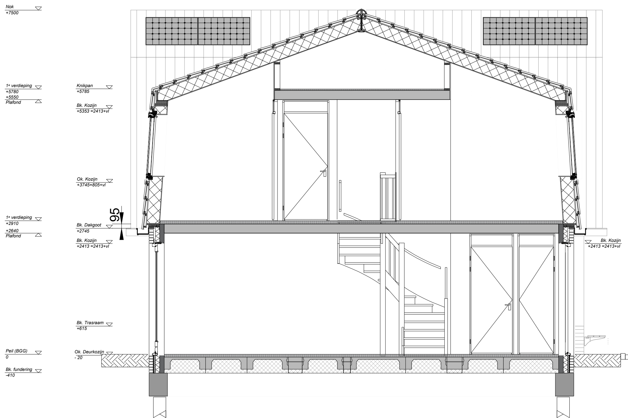
Doorsnede tussenwoningen
