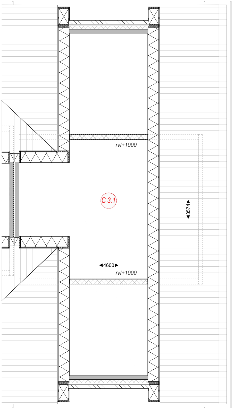
Vliering
