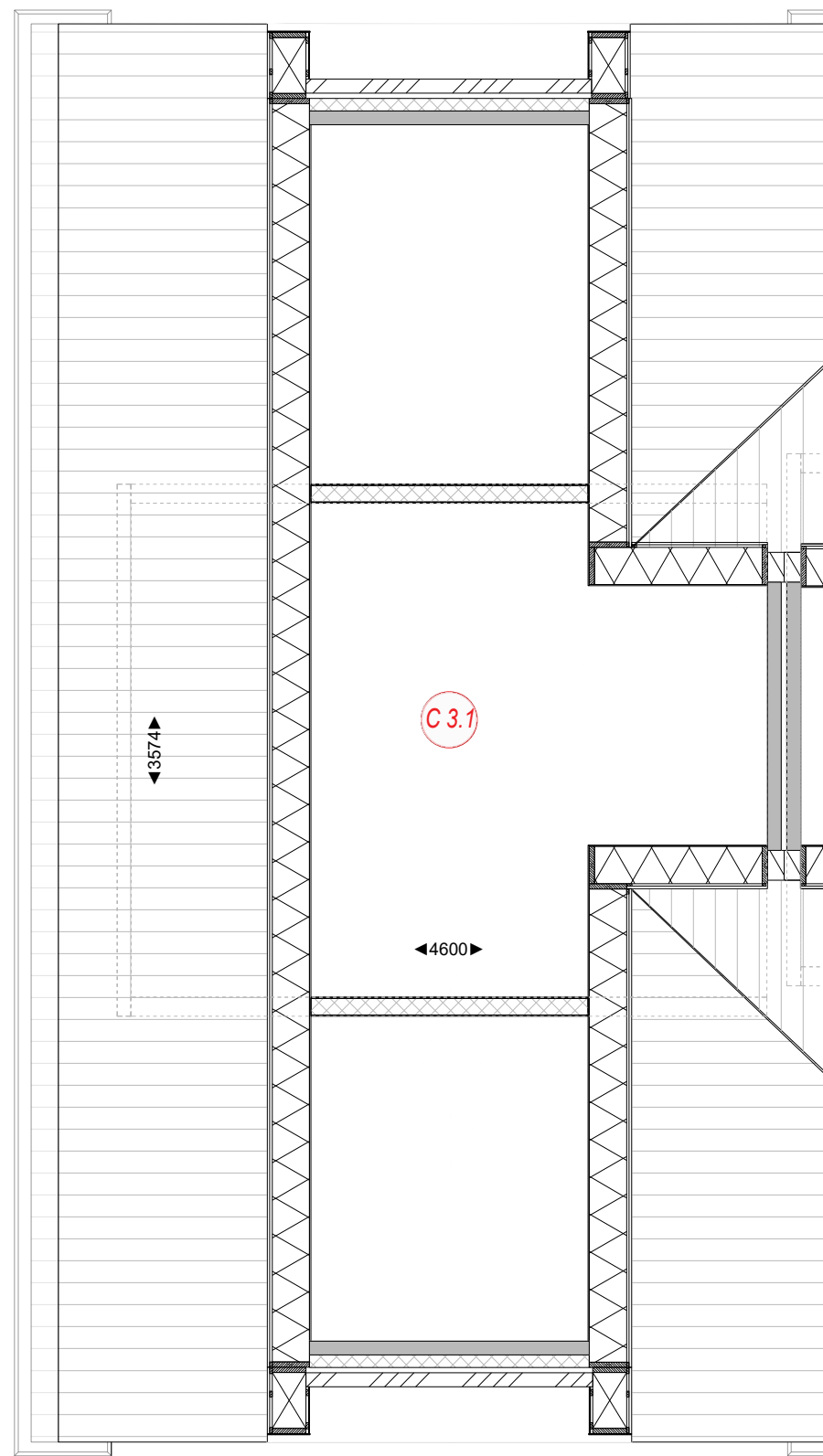
Vliering
