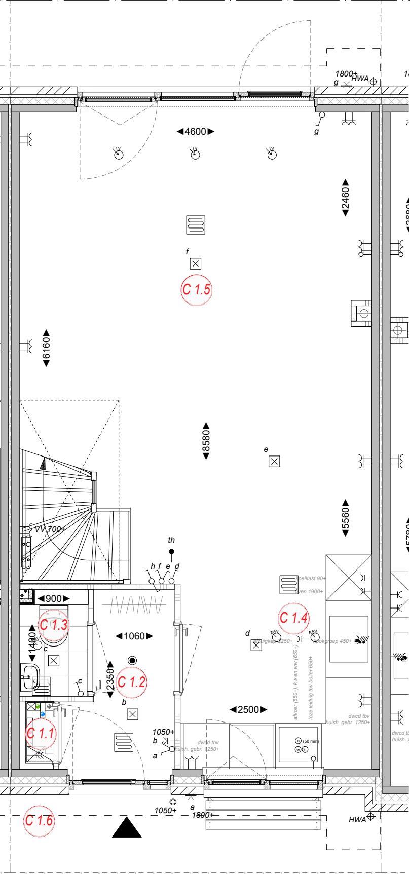
Begane grond
