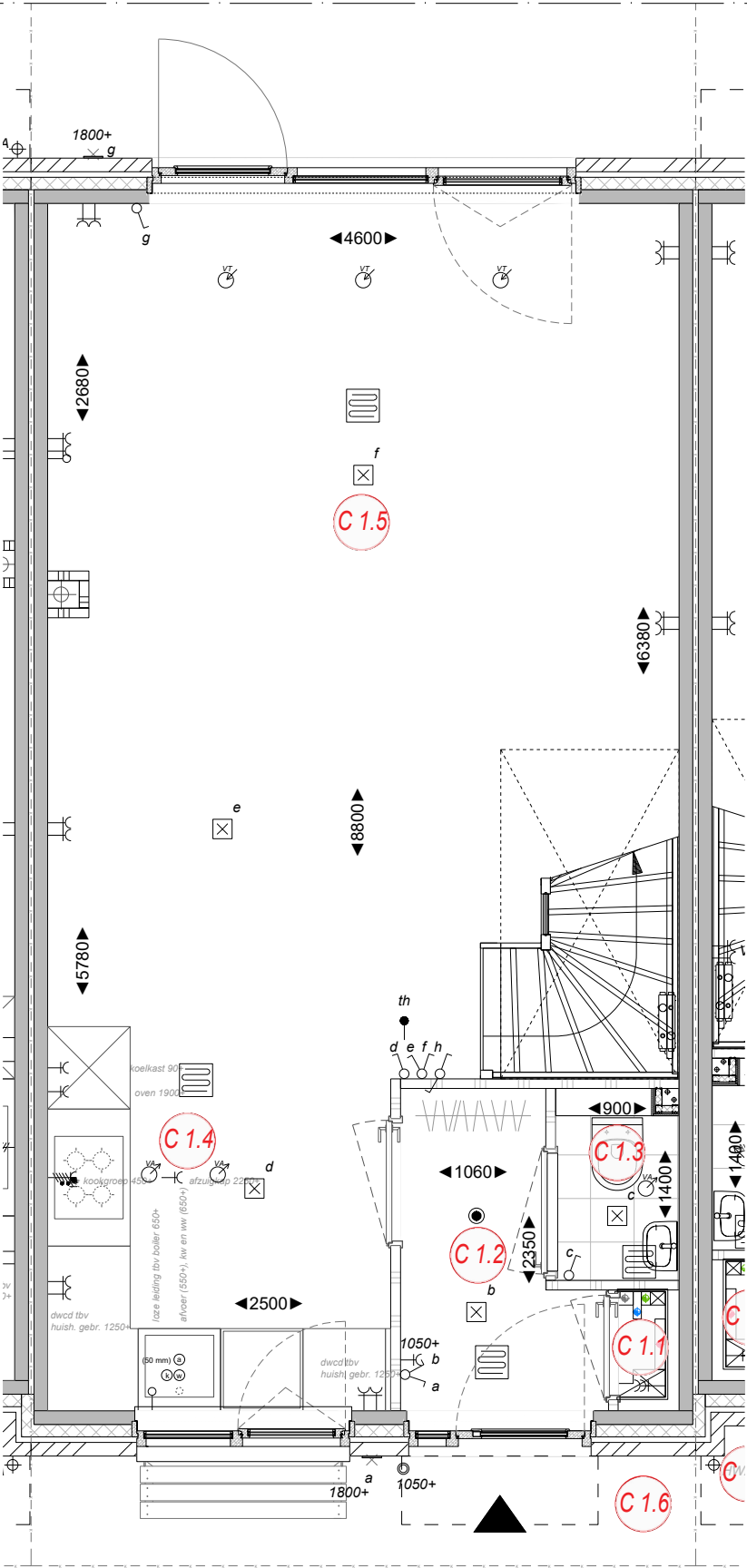
Begane grond
