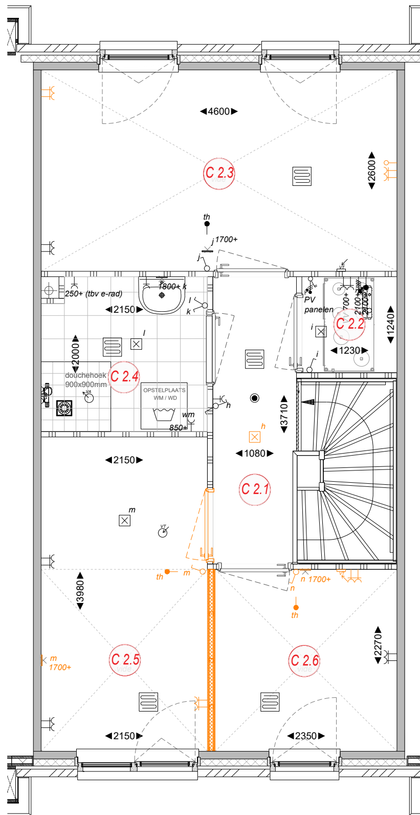
Kopwoning
