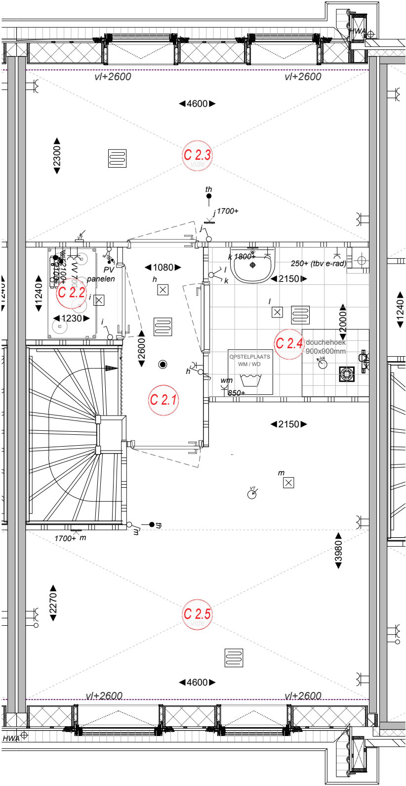
Eerste verdieping
