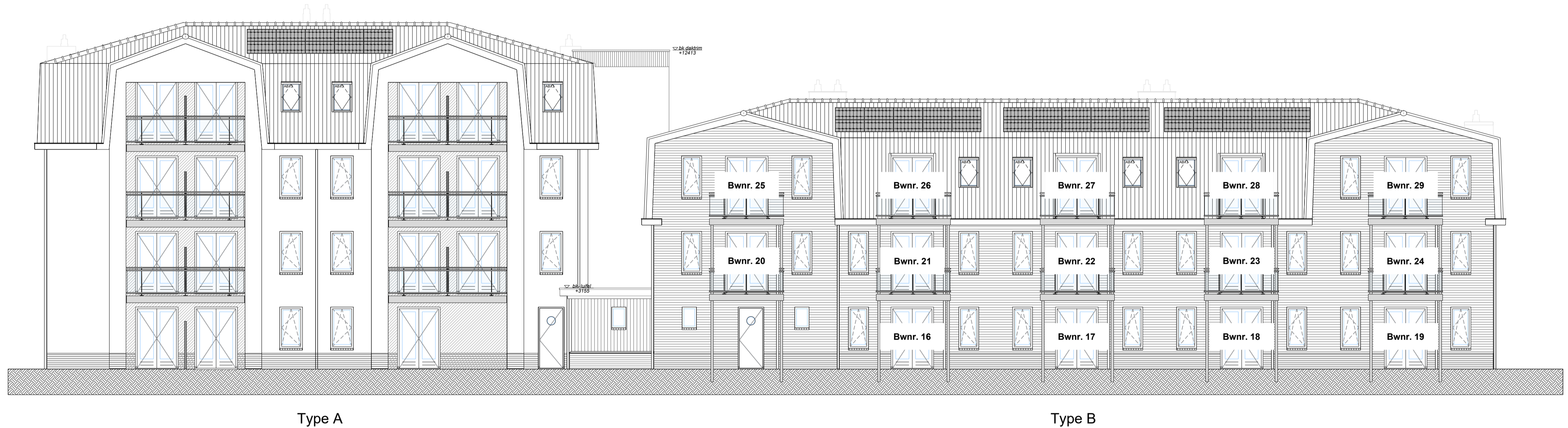
Achtergevel
