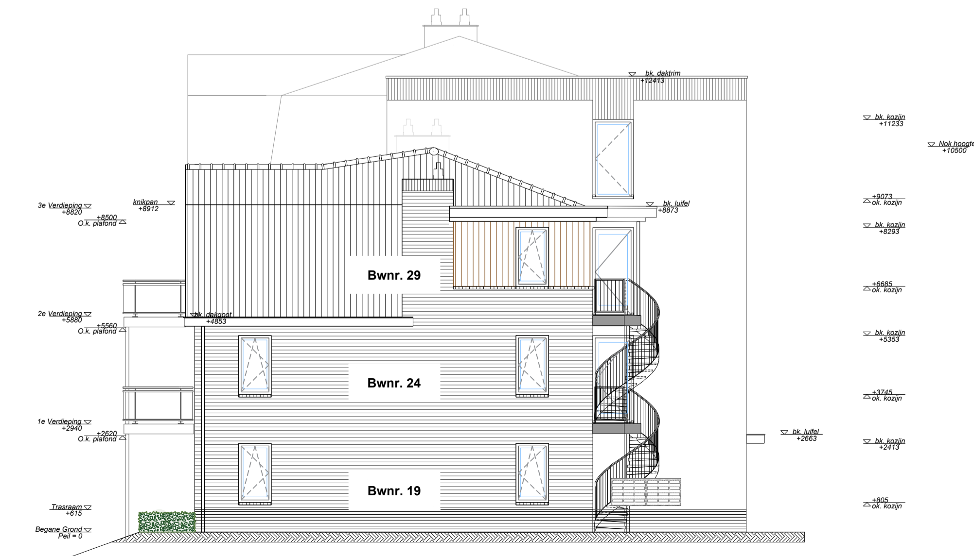
Zijgevel
